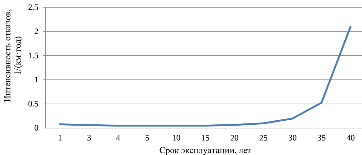
Рис. 2.1.5 – Интенсивность отказов в зависимости от срока эксплуатации участка тепловой сети
