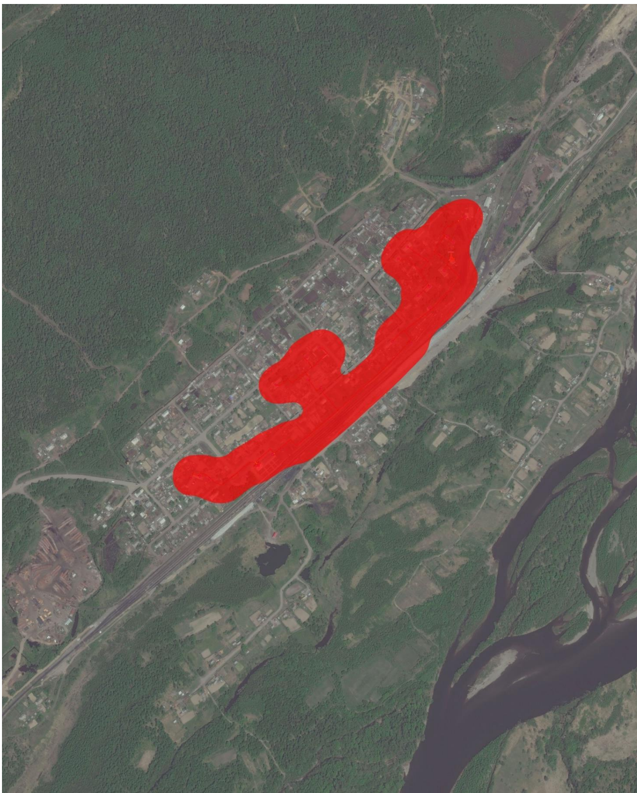
Рис. 2.1.1 – Зона действия системы теплоснабжения п. Тумнин.
