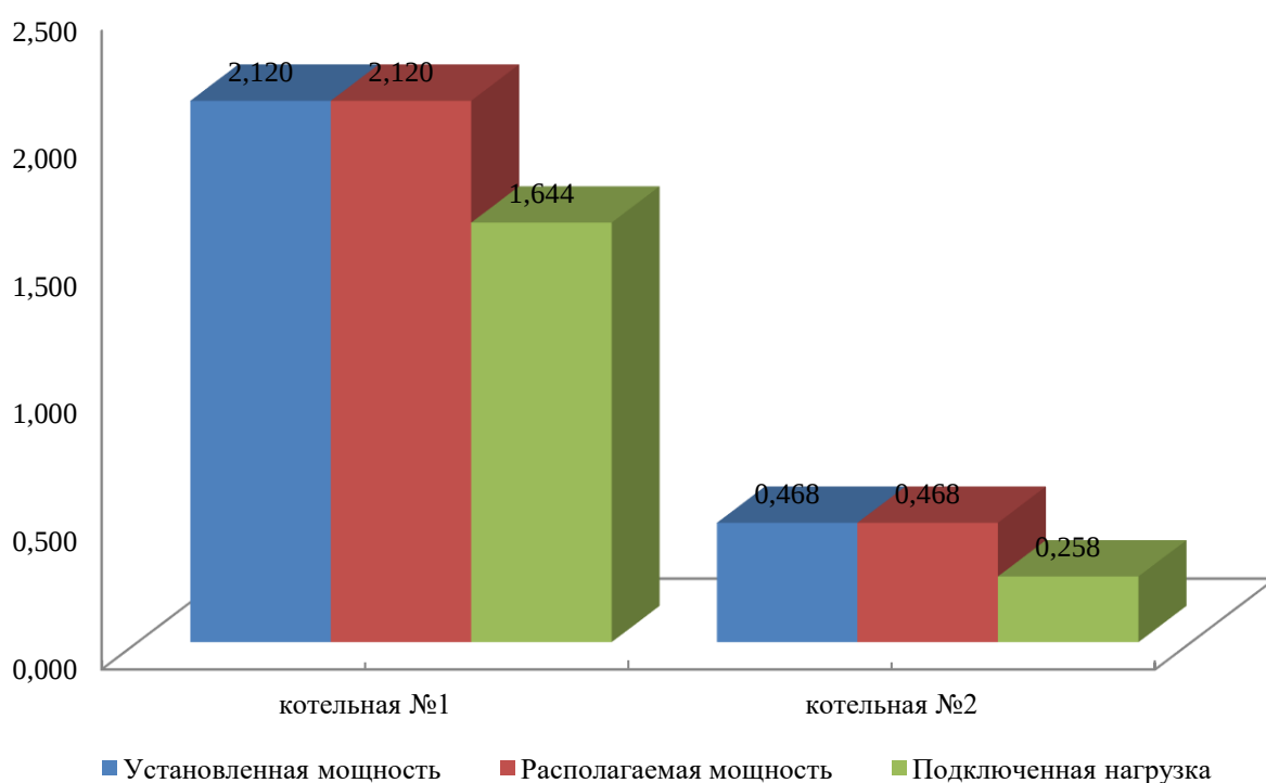
Рис. 2.1.2 – Распределение мощностей источников тепловой энергии
